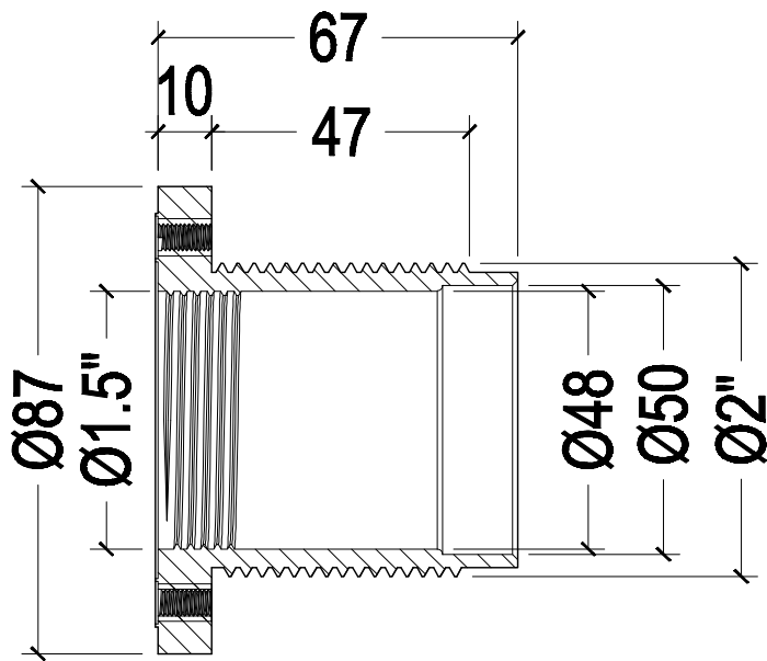
剖面图
