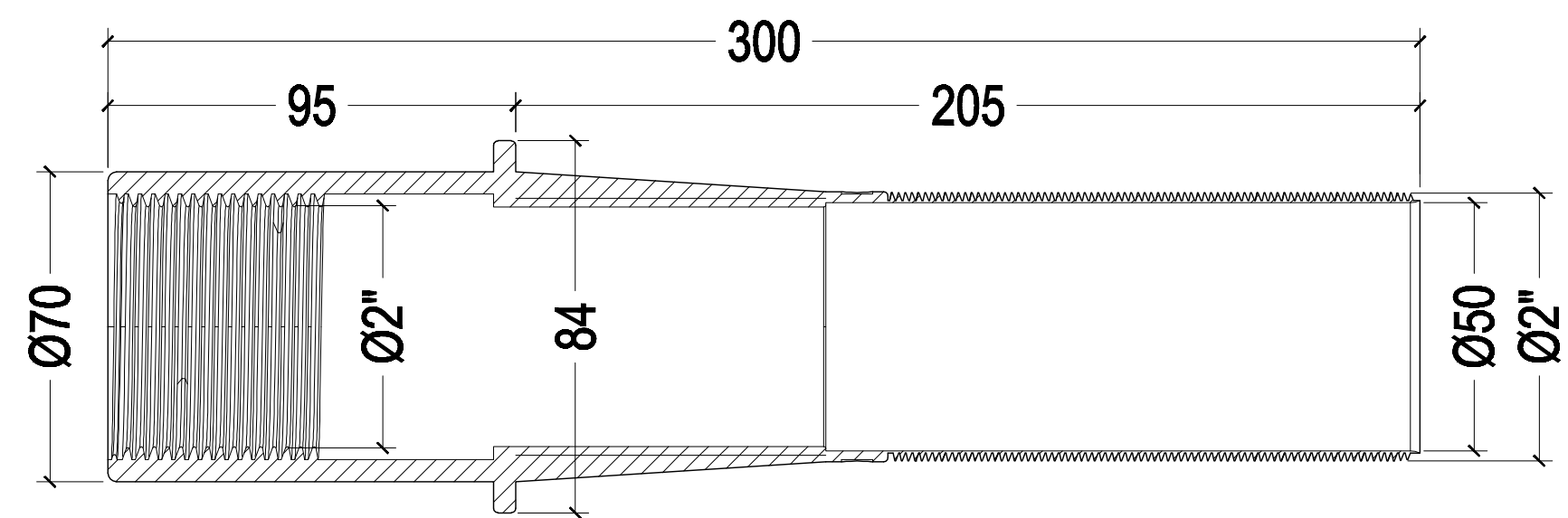
剖面图
