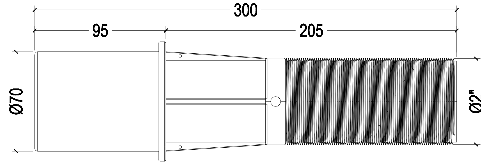
剖面图
